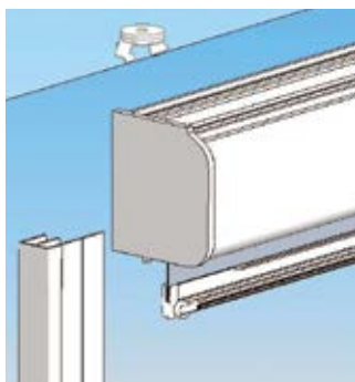
Mit Deckenträgern
