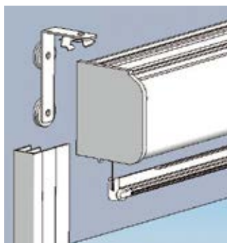
Mit Wandwinkeln
